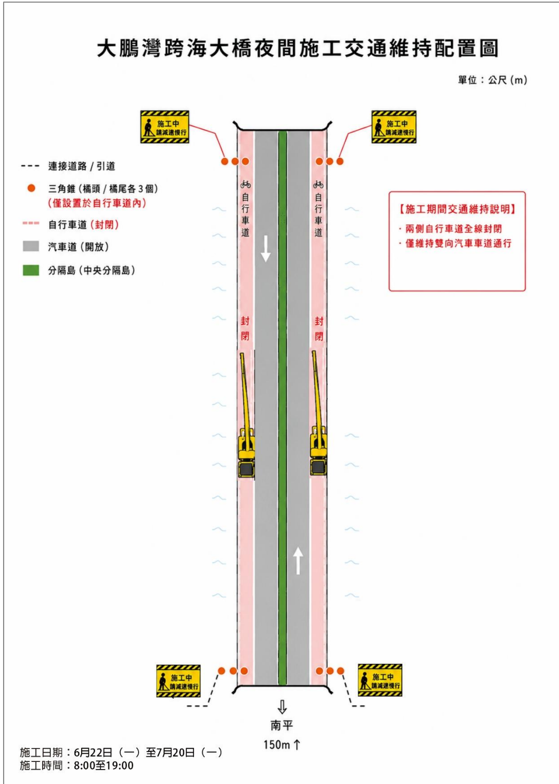
圖 2 鵬灣跨海大橋施工交維配置示意圖-自行車道側欄杆區域燈具拆除移動施工作業
