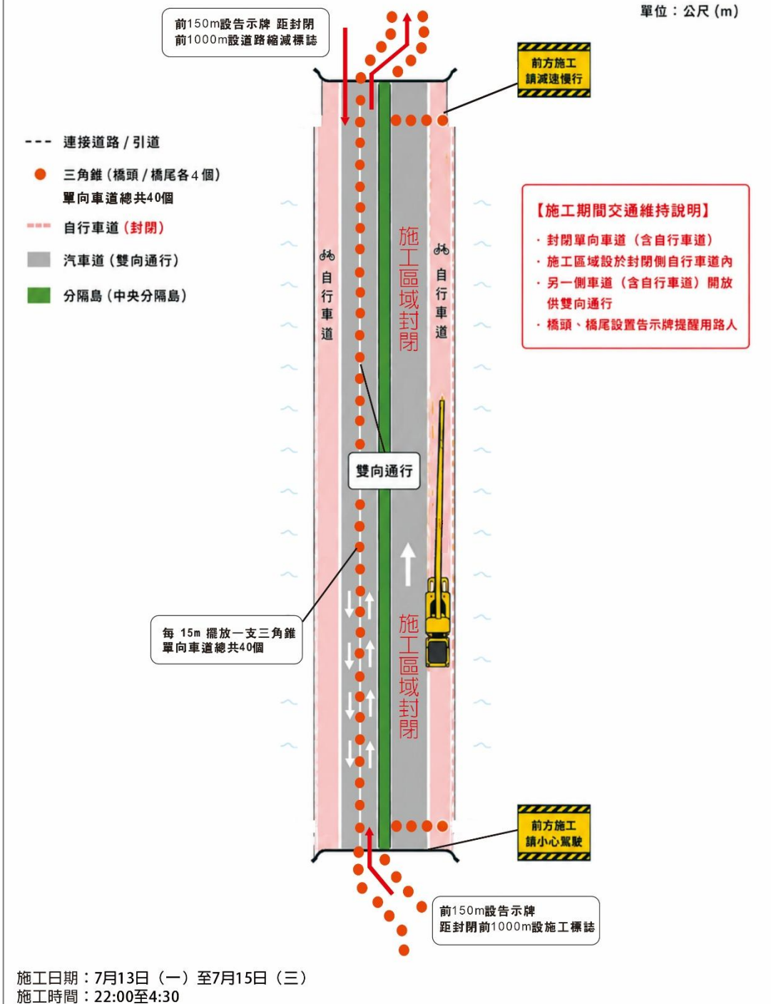
圖 3 鵬灣跨海大橋施工交維配置示意圖-橋面燈具吊掛拆除移動施工作業
